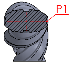
D-D (2 : 1)
